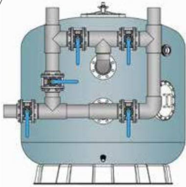
Povratna baterija Backwash Battery
