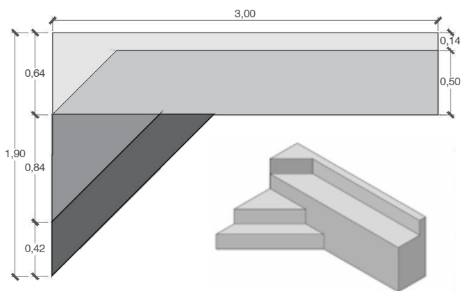
šifra.1030410 (br.2 stepenika) - šifra. 1030413 (br.1 stepenika)
