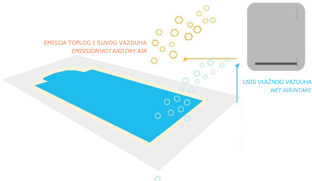
Fig 8: Funkcionisanje odvlaživača
