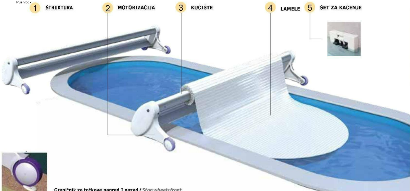
Graničnik za točkove napred i nazad / Stop wheels front
