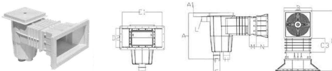
SKIMMER SA PROŠIRENIM OTVOROM SA PRODUŽETKOM / WIDE MOUTH SKIMMER WITH EXTENSION
