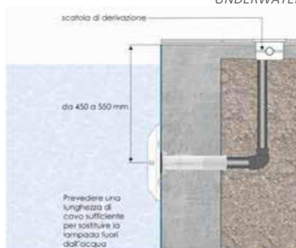
REFLEKTOR UNDERWATER LIGHT
