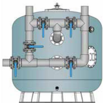
BATERIJE ZA POVRATNO ISPIRANJE BACKWASH BATTERIES
